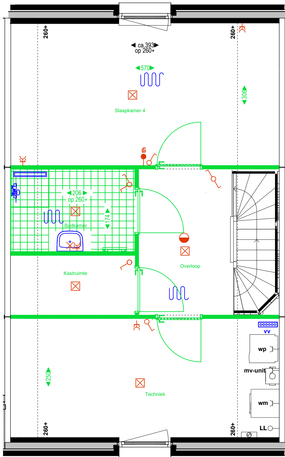
2e verdieping
