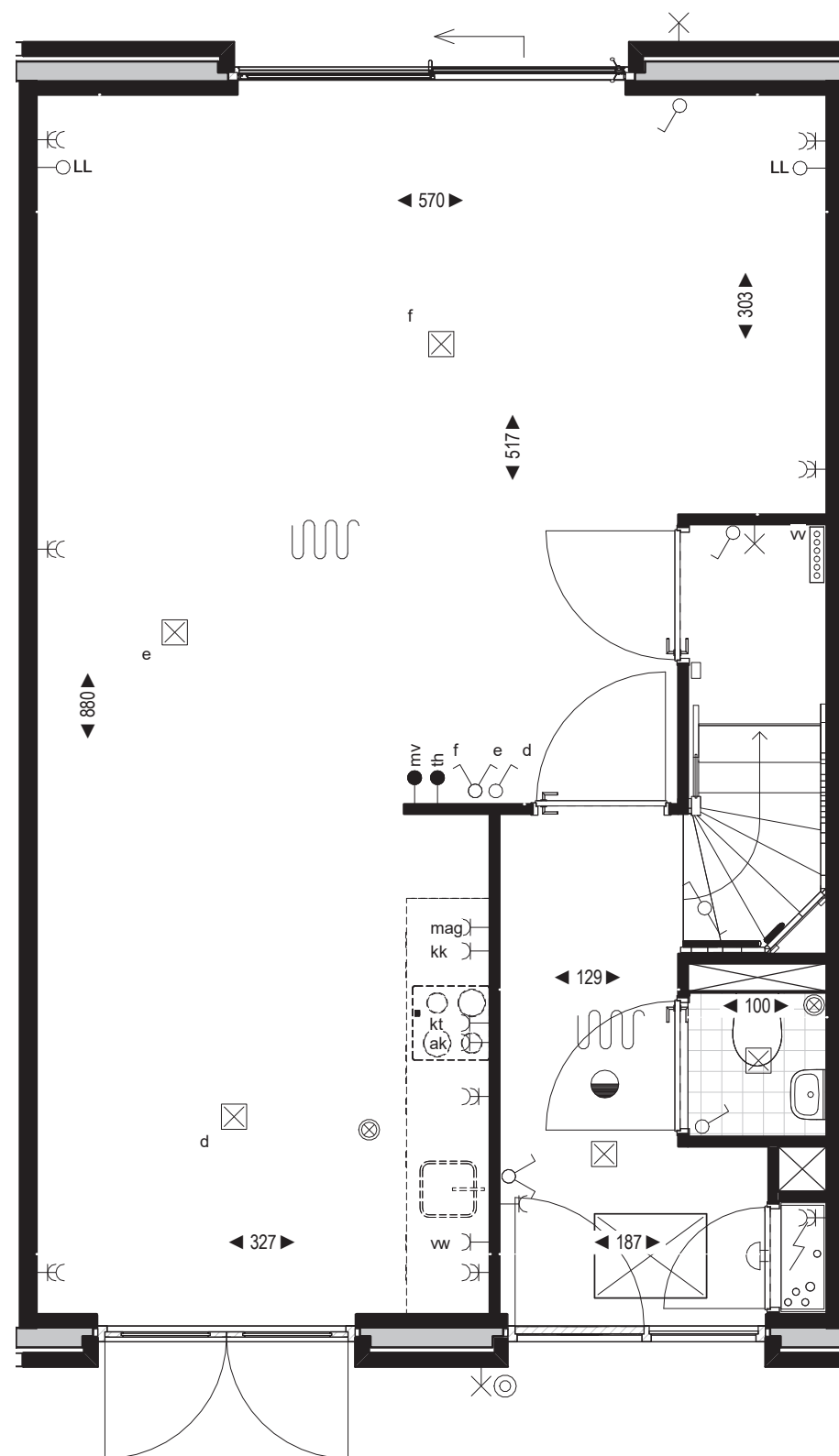
Begane grond bouwnummer 40 Woningtype F
