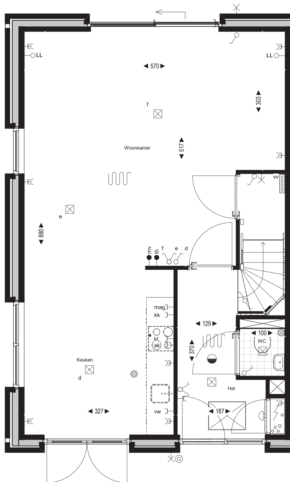
Begane grond bouwnummer 38 Woningtype F
