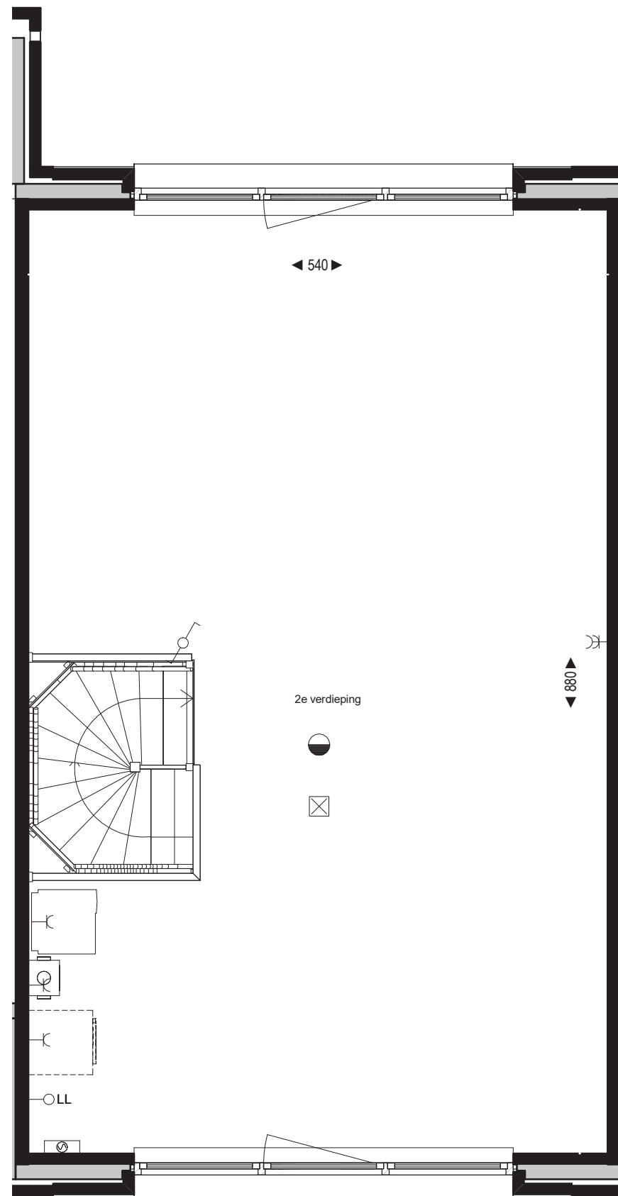
Tweede verdieping bouwnummer 42 Woningtype D
