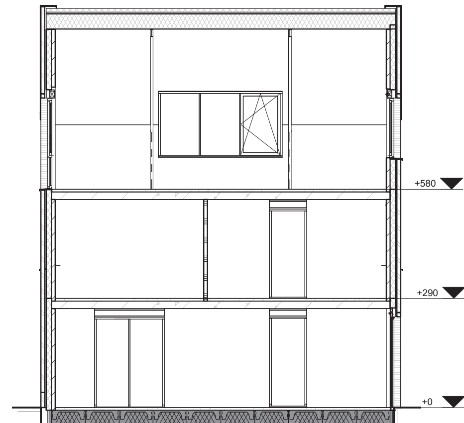
Doorsnede Woningtype F
