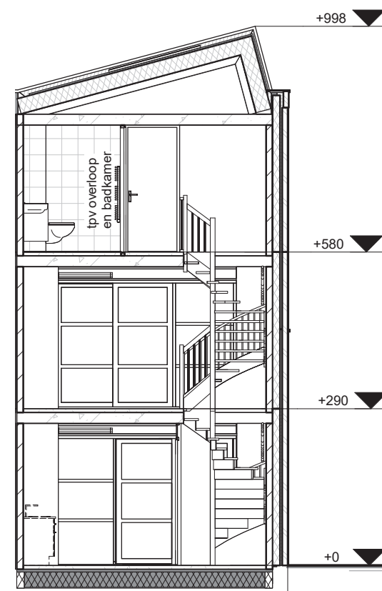
Doorsnede Woningtype C
