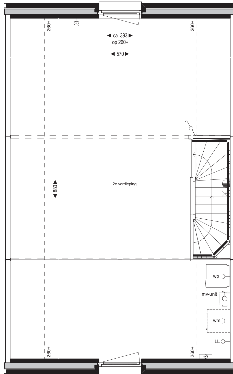
Tweede verdieping bouwnummer 39 Woningtype F
