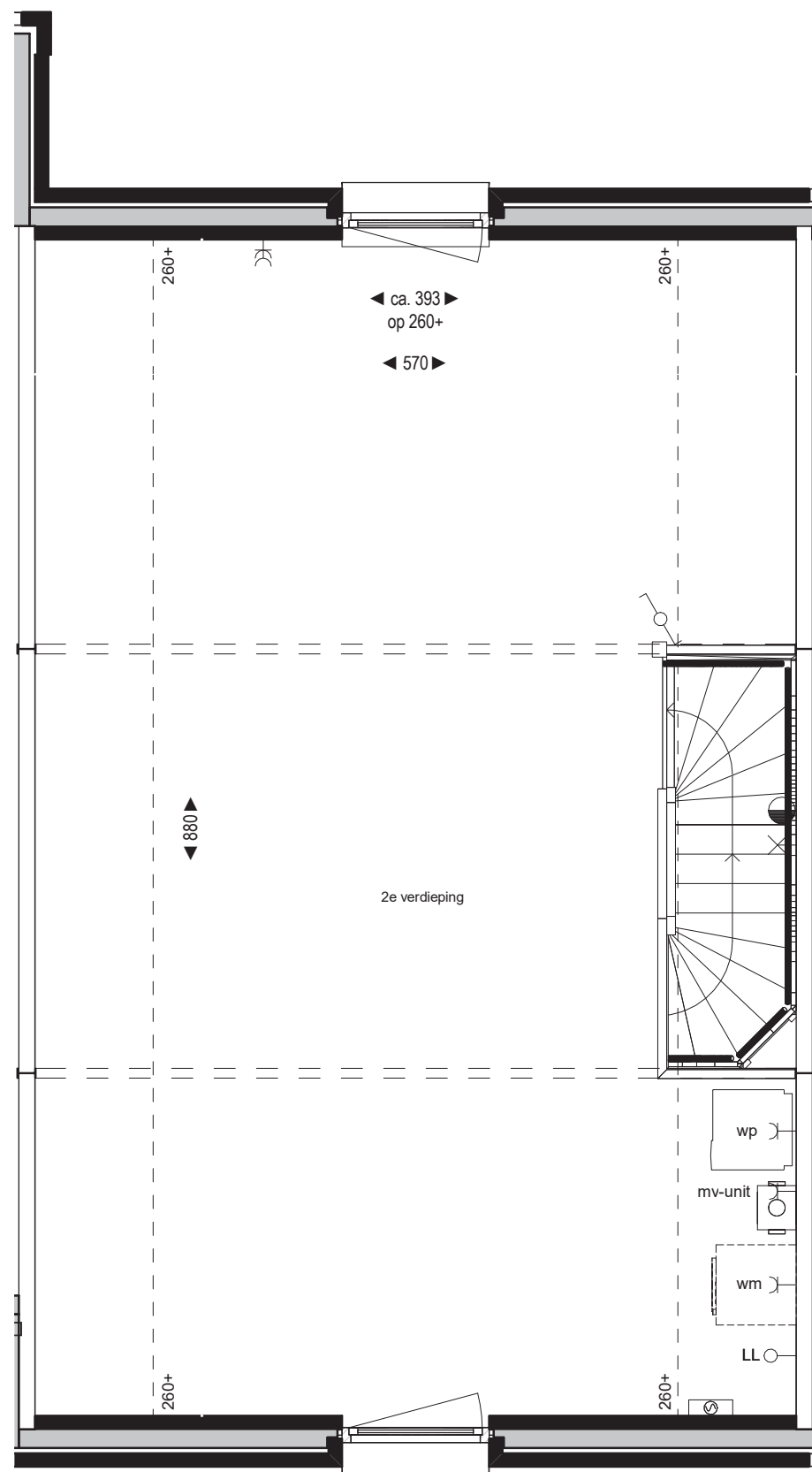
Tweede verdieping bouwnummer 13 Woningtype F
