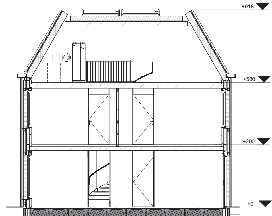
Doorsnede Woningtype E
