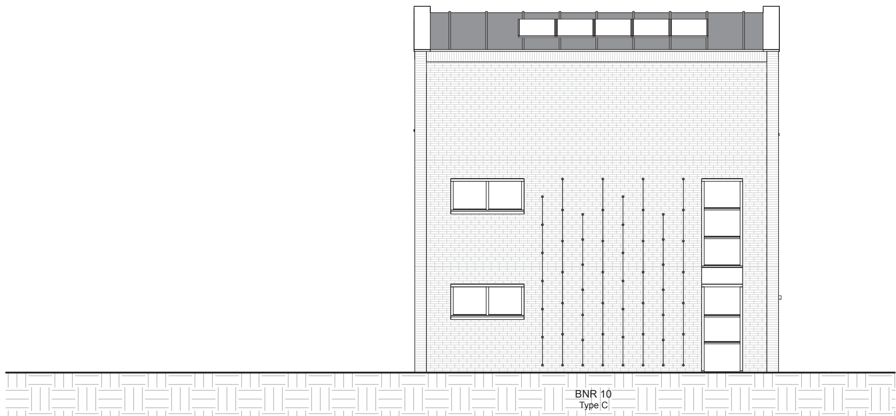
Linker gevel
