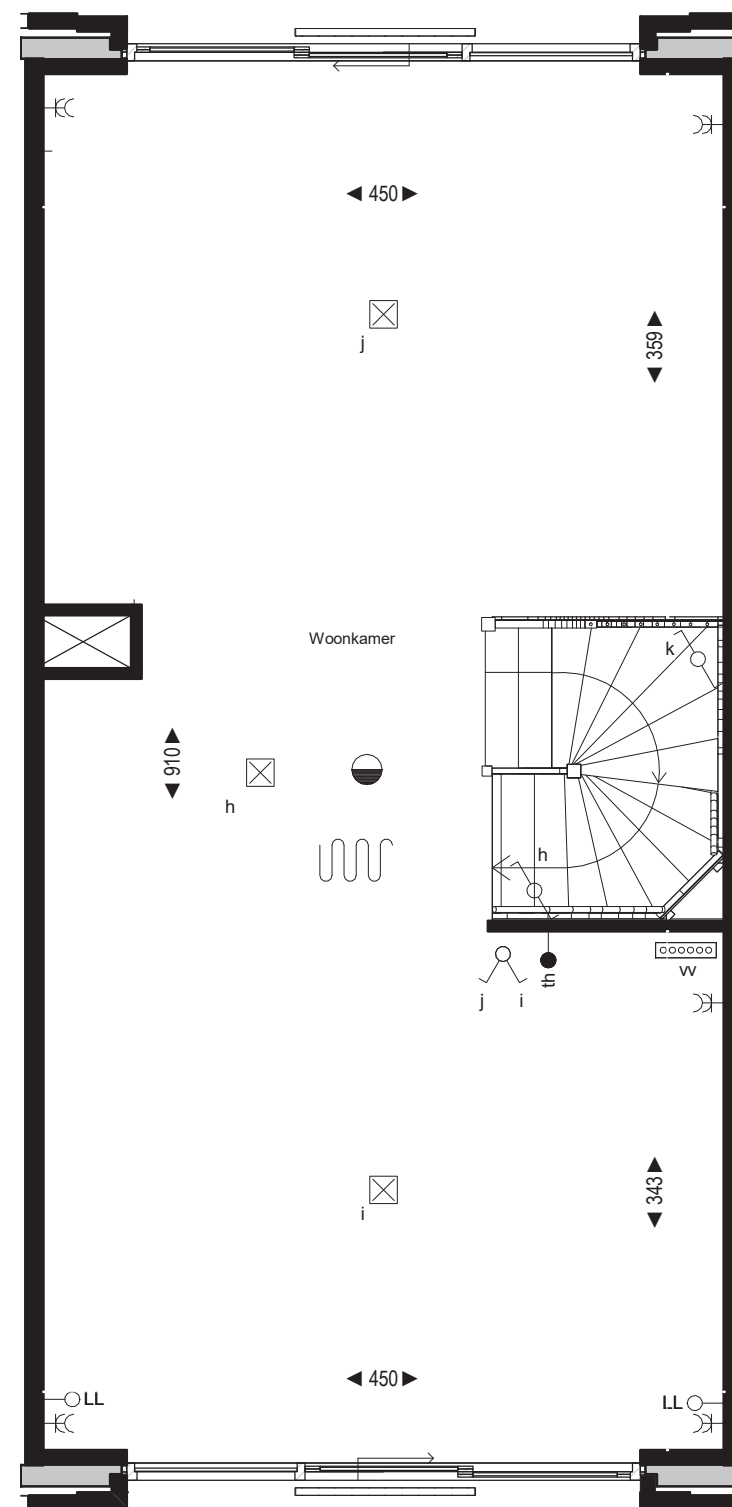
1e verdieping grond bouwnummer 11 Woningtype C
