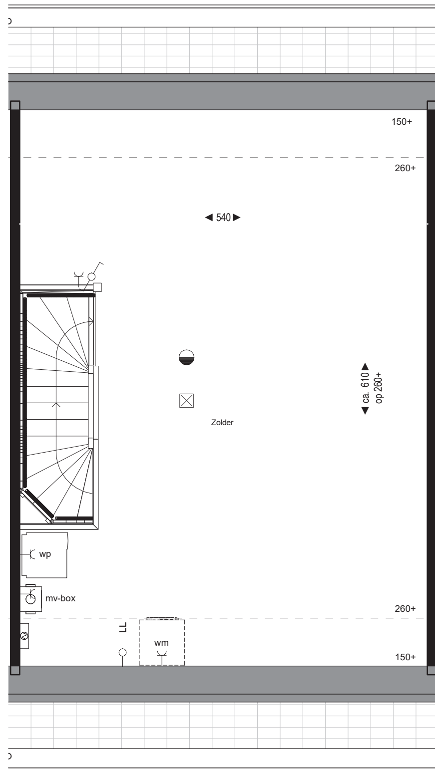
Tweede verdieping bouwnummer 16 Woningtype E
