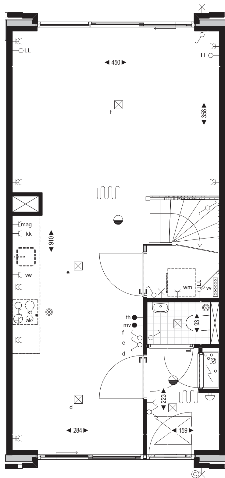
Begane grond bouwnummer 44 Woningtype C
