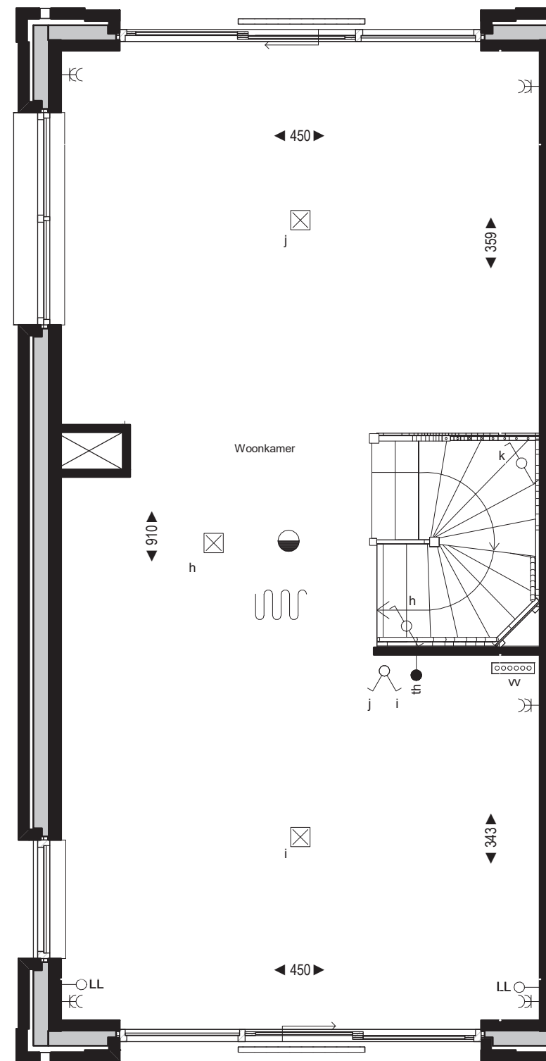
1e verdieping grond bouwnummer 10 Woningtype C
