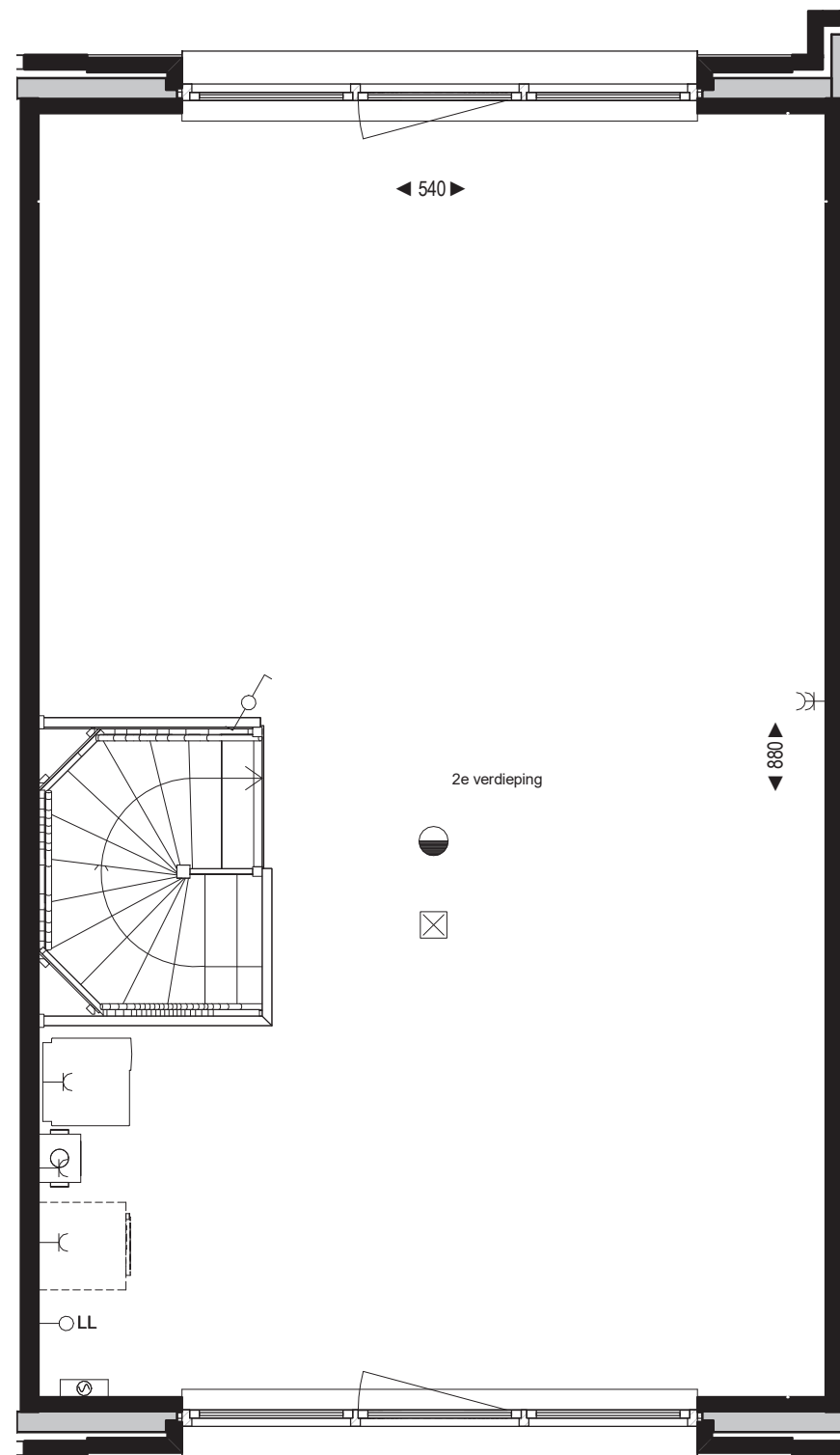
Tweede verdieping bouwnummer 43 Woningtype D
