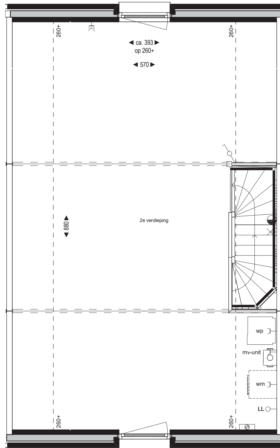
Tweede verdieping bouwnummer 40 Woningtype F
