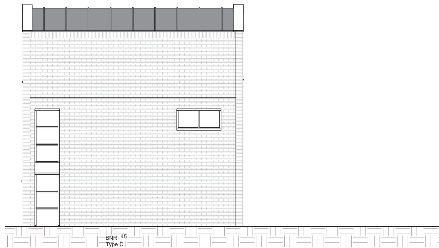
Rechter gevel
