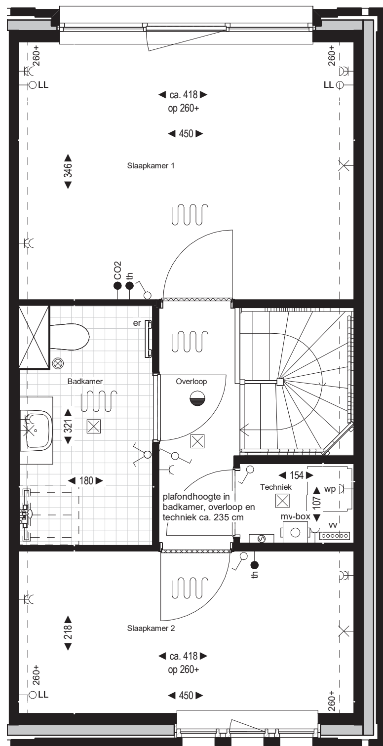
Tweede bouwnummer 45 Woningtype C
