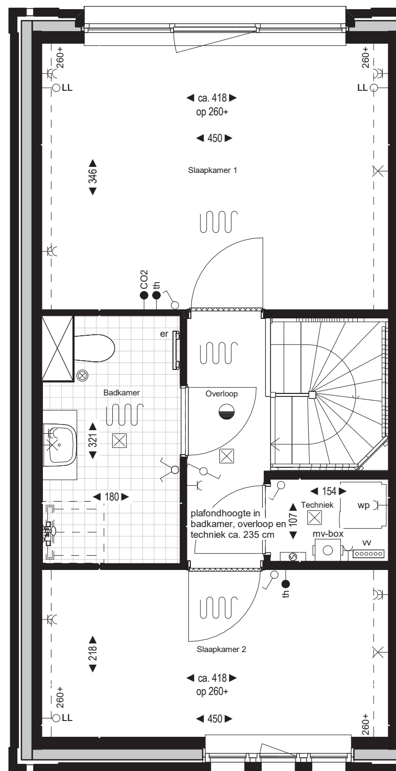
Tweede verdieping bouwnummer 10 Woningtype C
