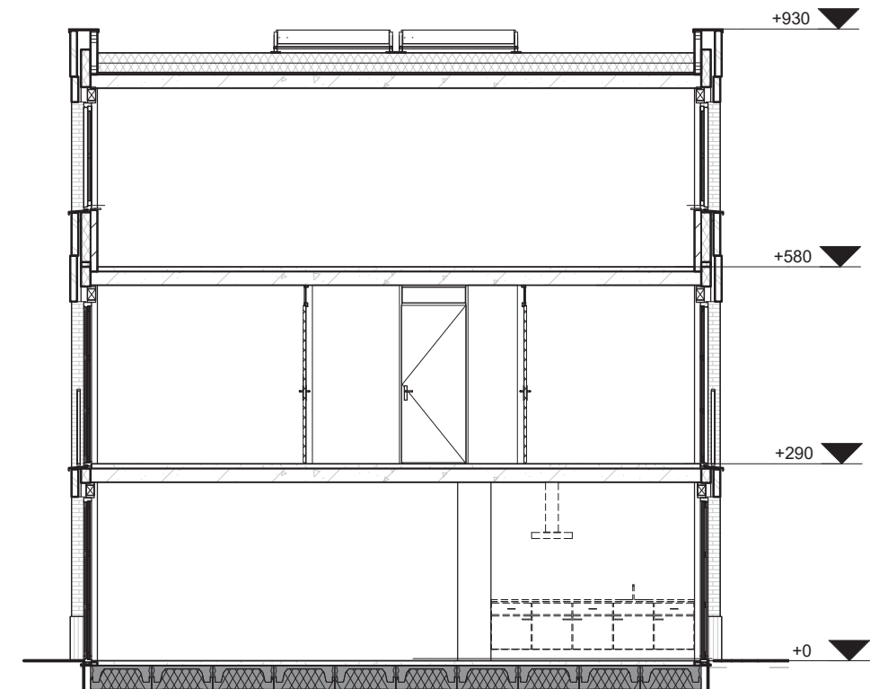
Doorsnede Woningtype D
