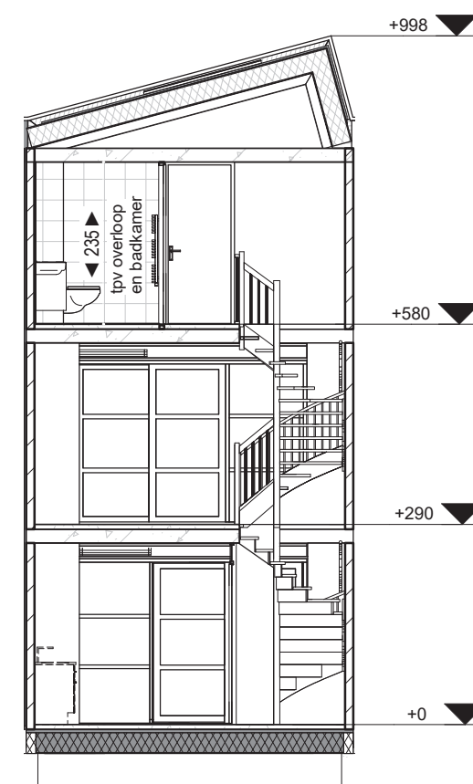
Doorsnede Woningtype C
