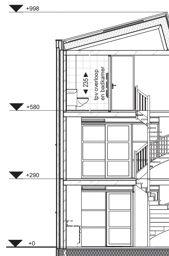
Doorsnede Woningtype C
