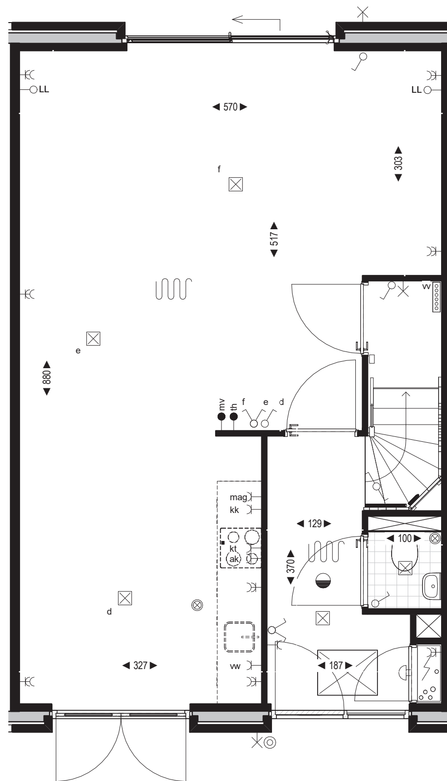
Begane grond bouwnummer 14 Woningtype F
