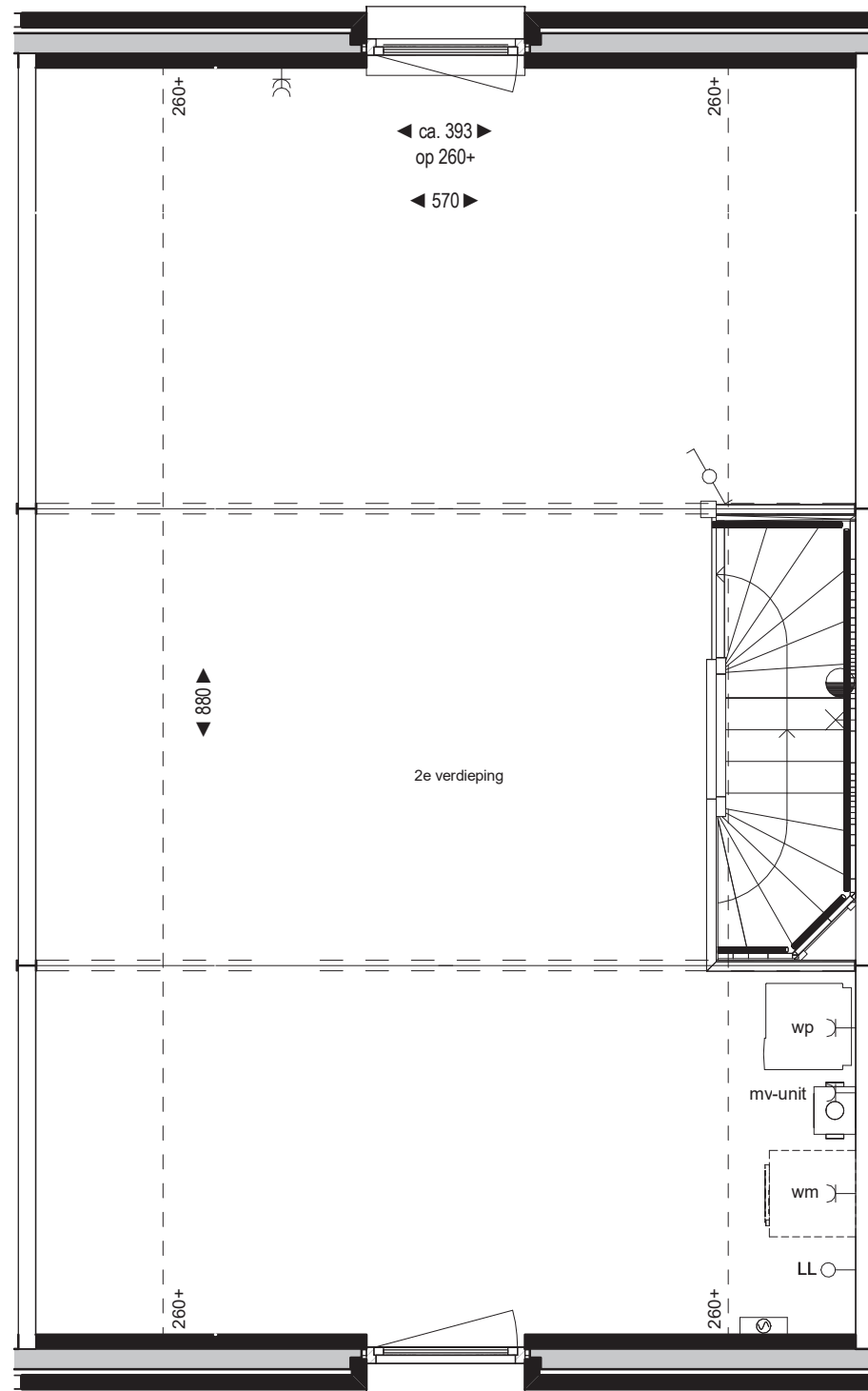
Tweede verdieping bouwnummer 14 Woningtype F
