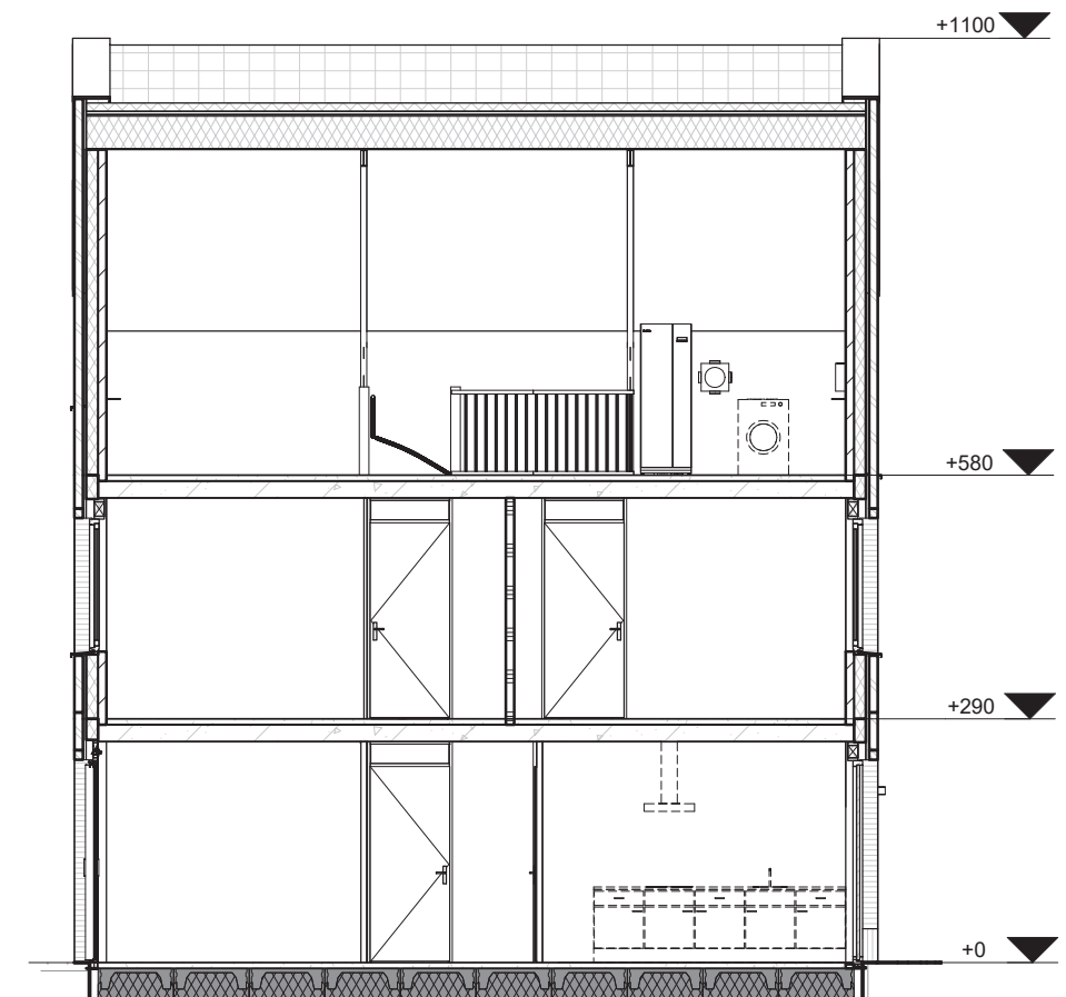
Doorsnede Woningtype F
