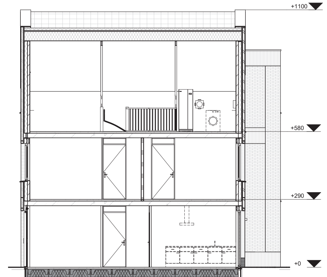
Doorsnede Woningtype F
