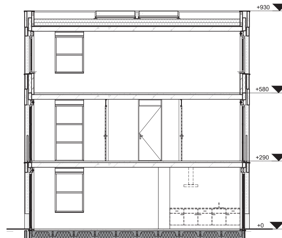
Doorsnede Woningtype D
