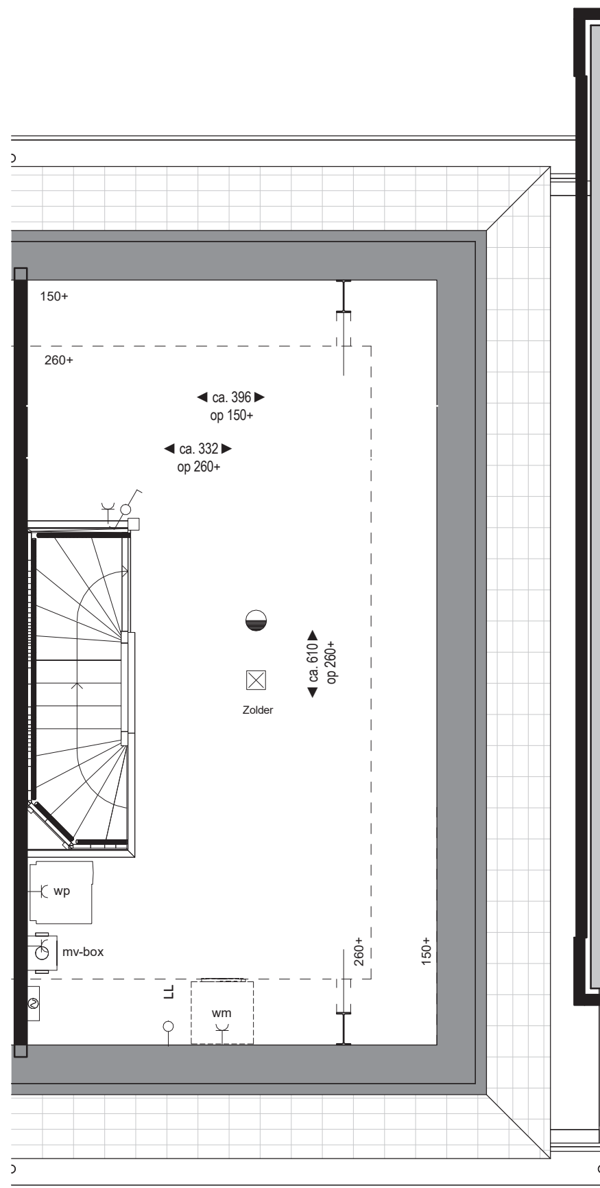
Tweede verdieping bouwnummer 17 Woningtype E
