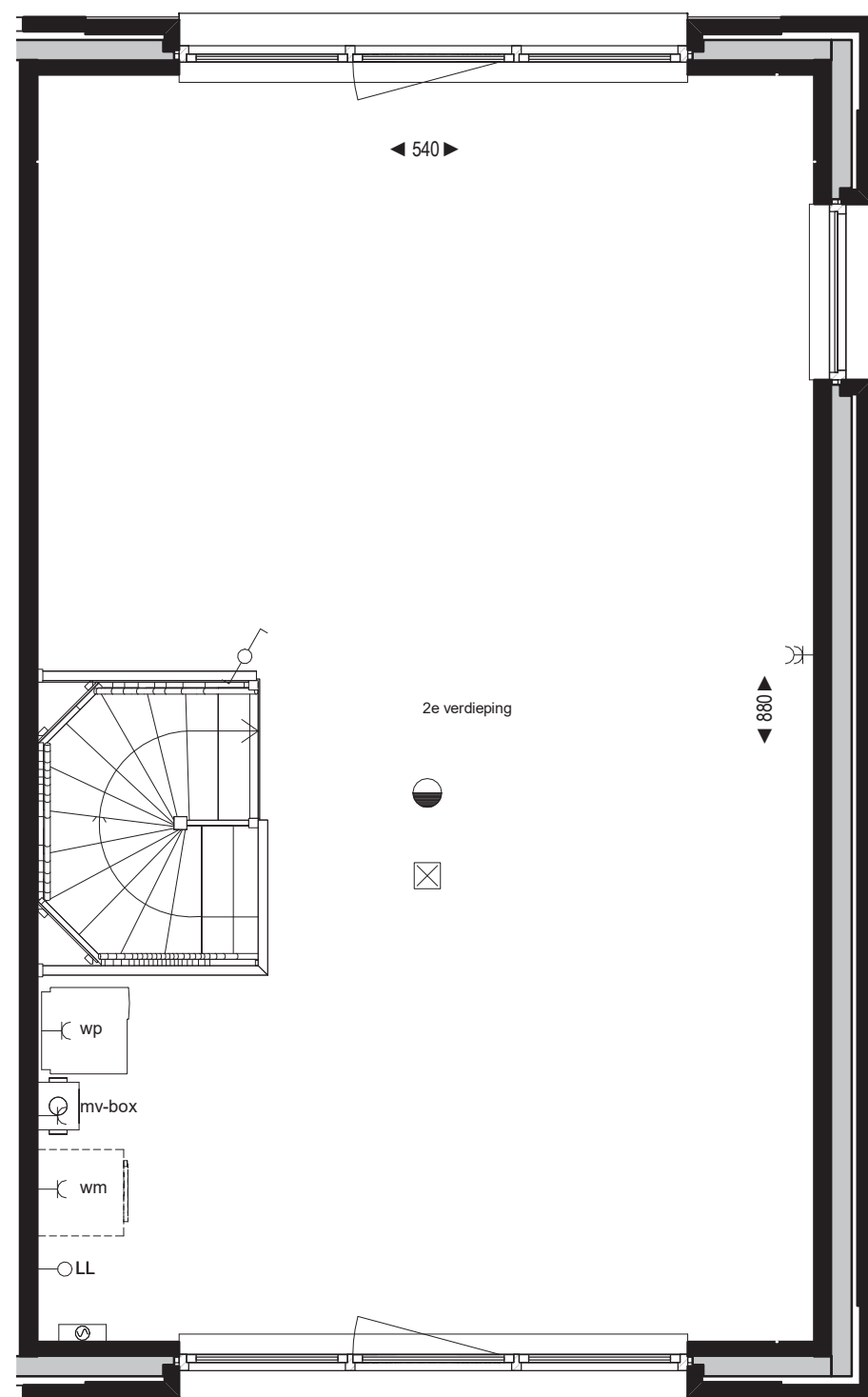
Tweede verdieping bouwnummer 19 Woningtype D
