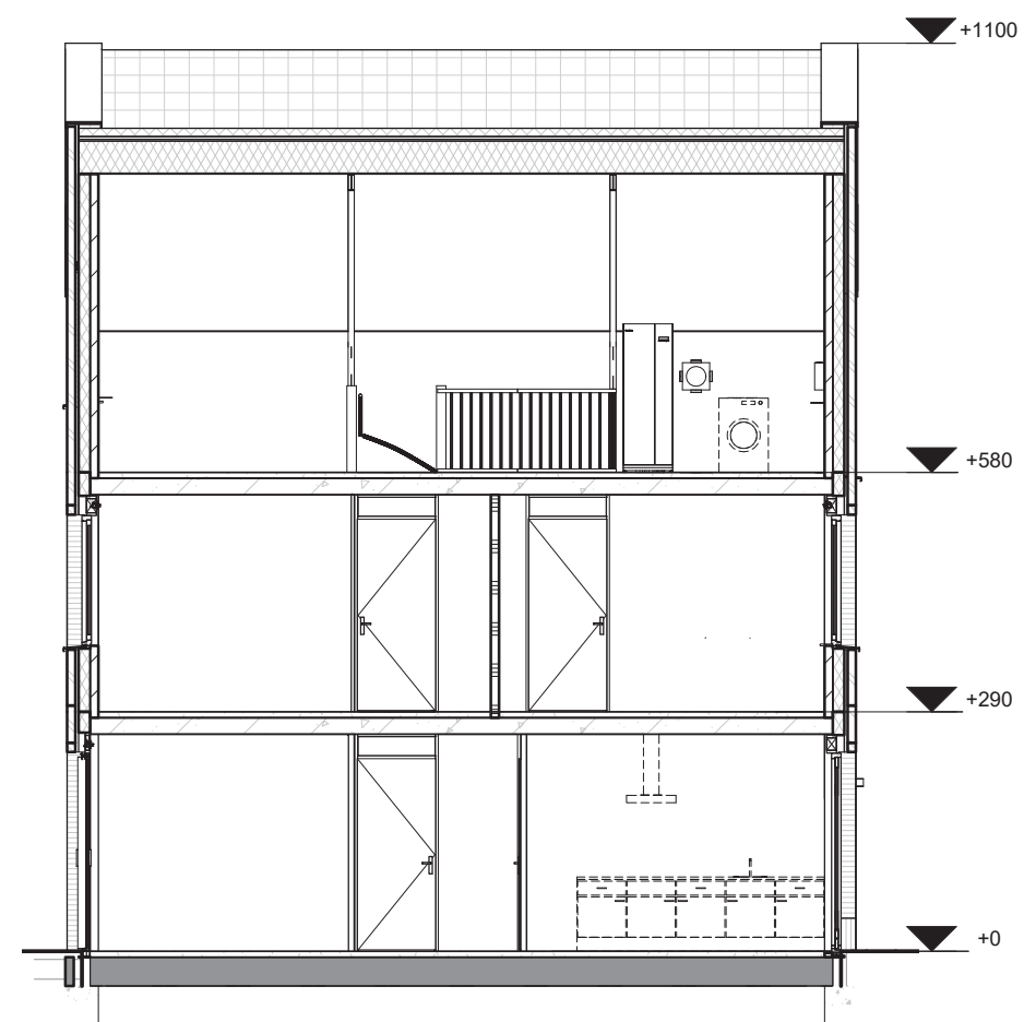
Doorsnede Woningtype F
