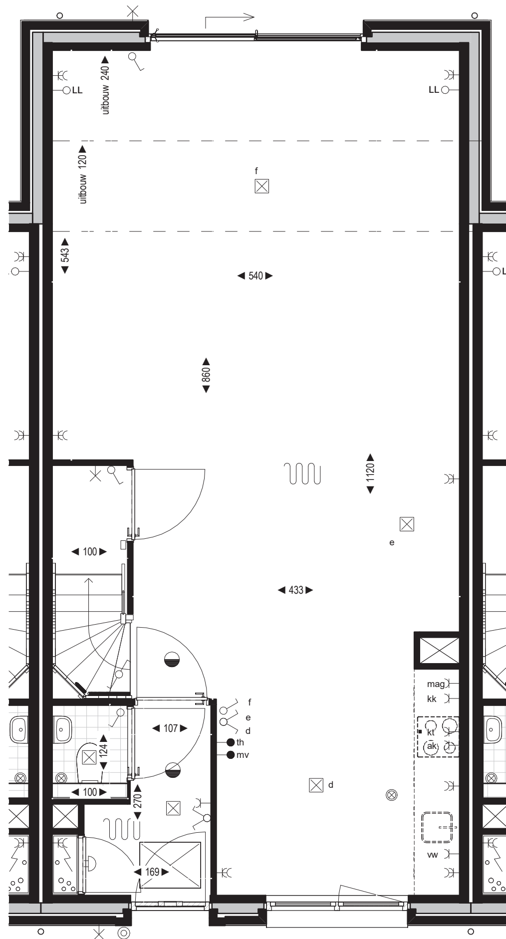
begane grond
