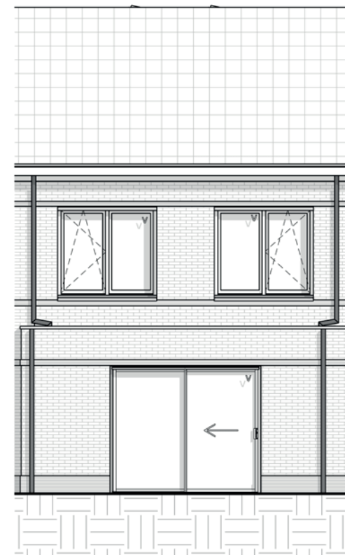
achtergevel
