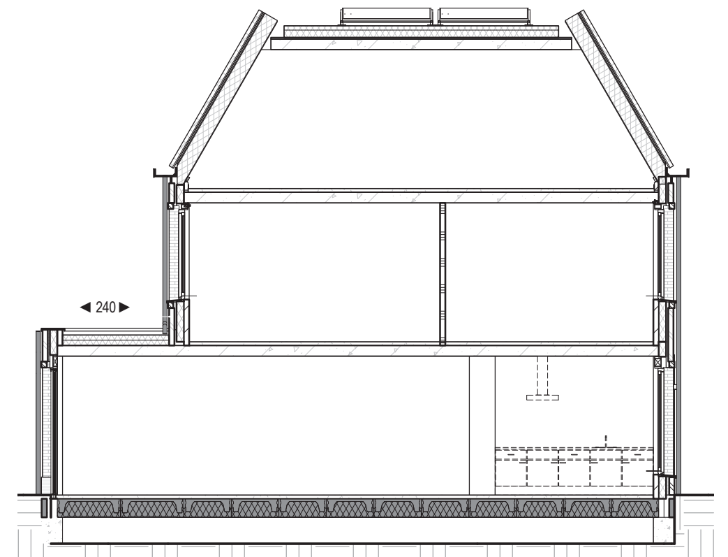
Doorsnede
