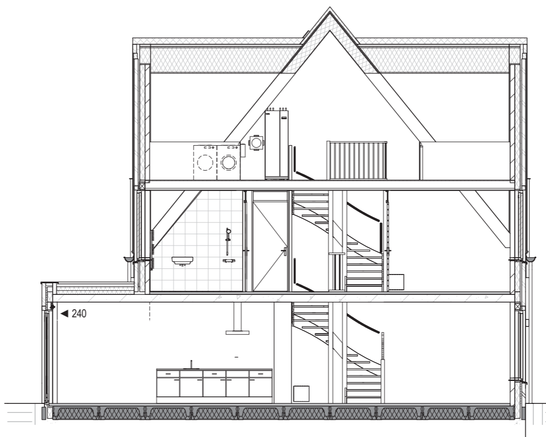
Doorsnede
