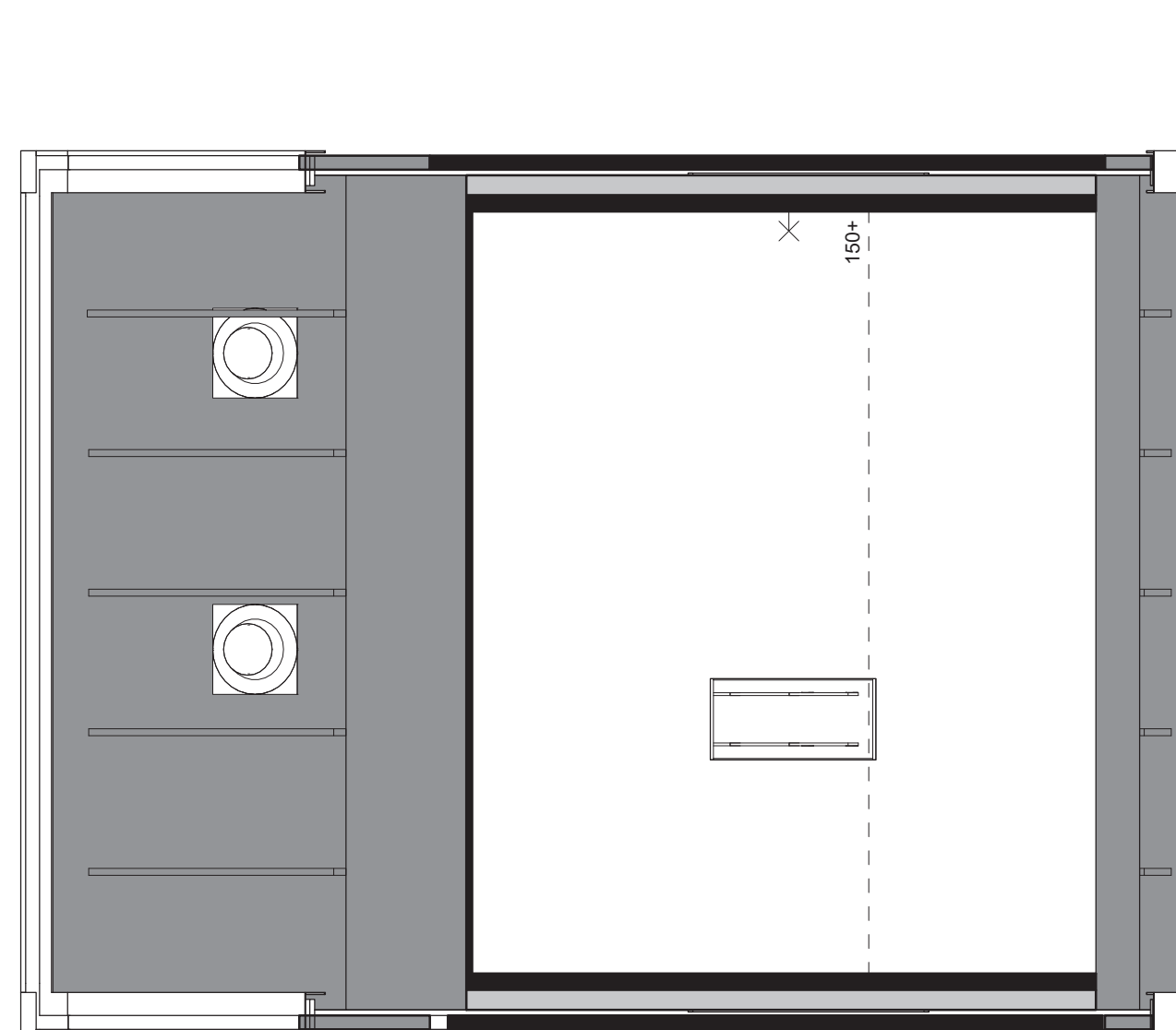
Vliering bouwnummer 27
