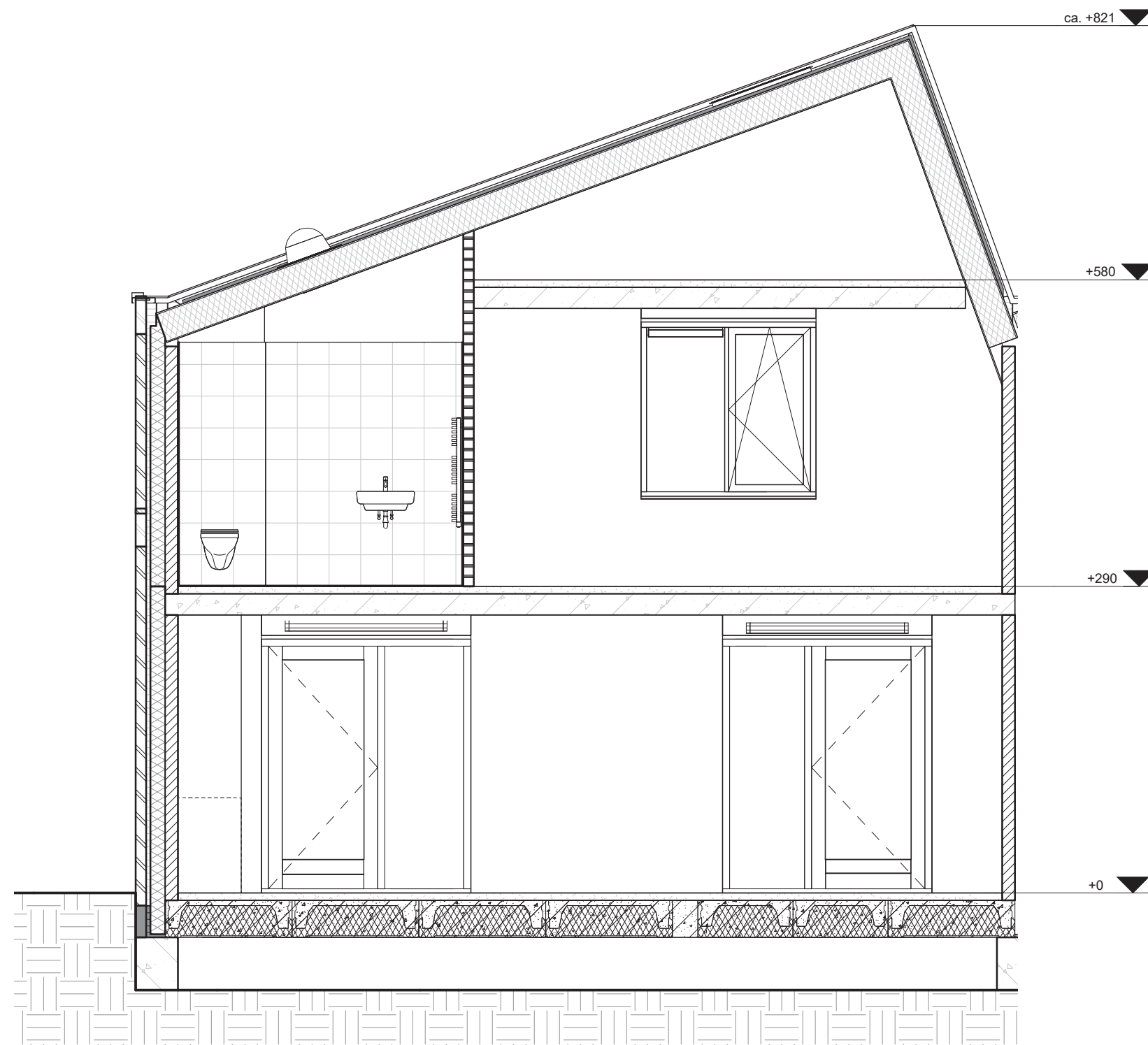
Doorsnede
