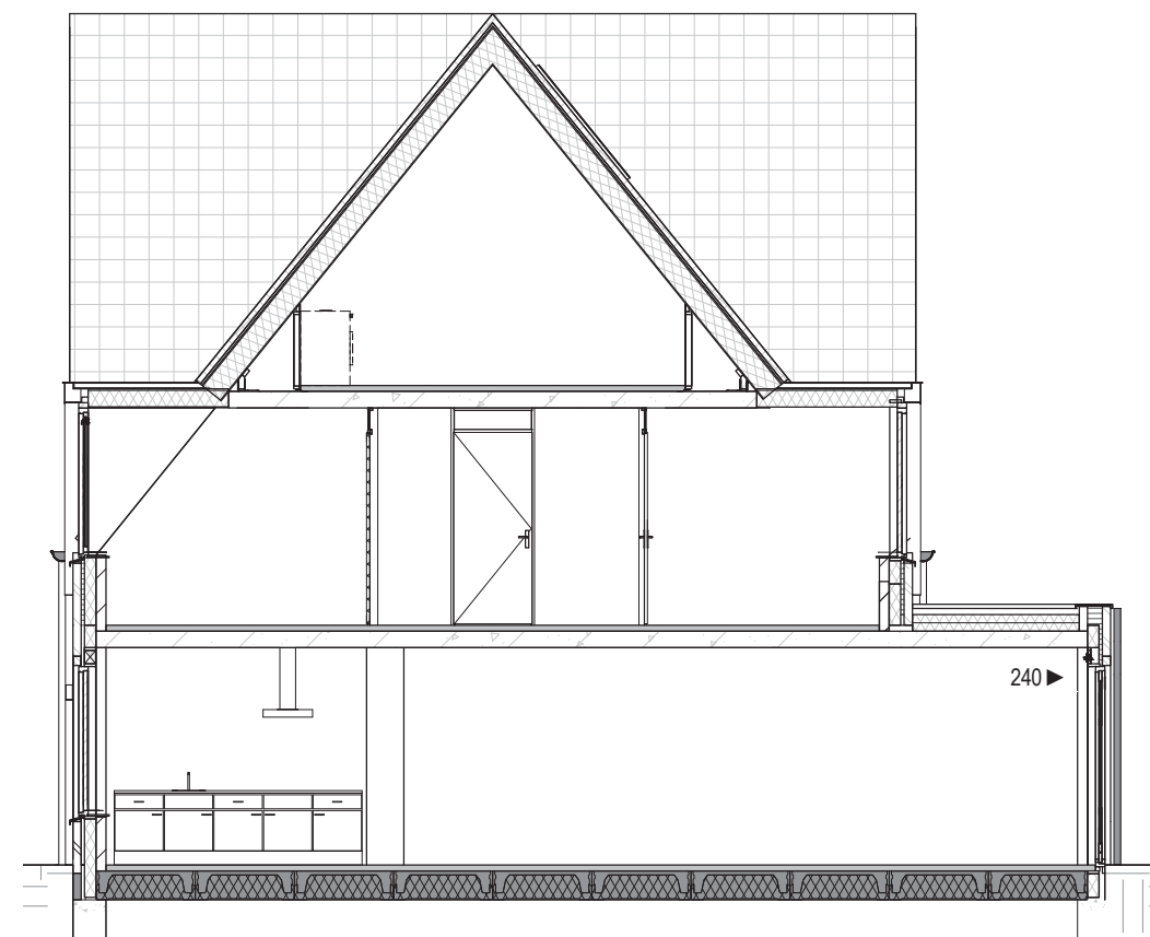
Doorsnede
