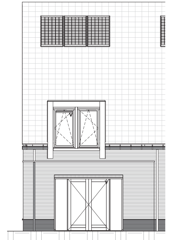
Bouwnummer 62 Achtergevel
