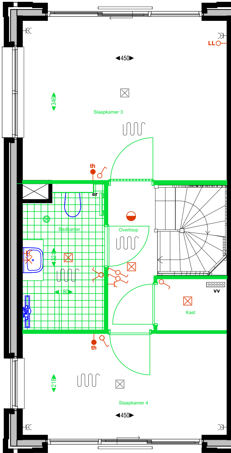
1e verdieping
