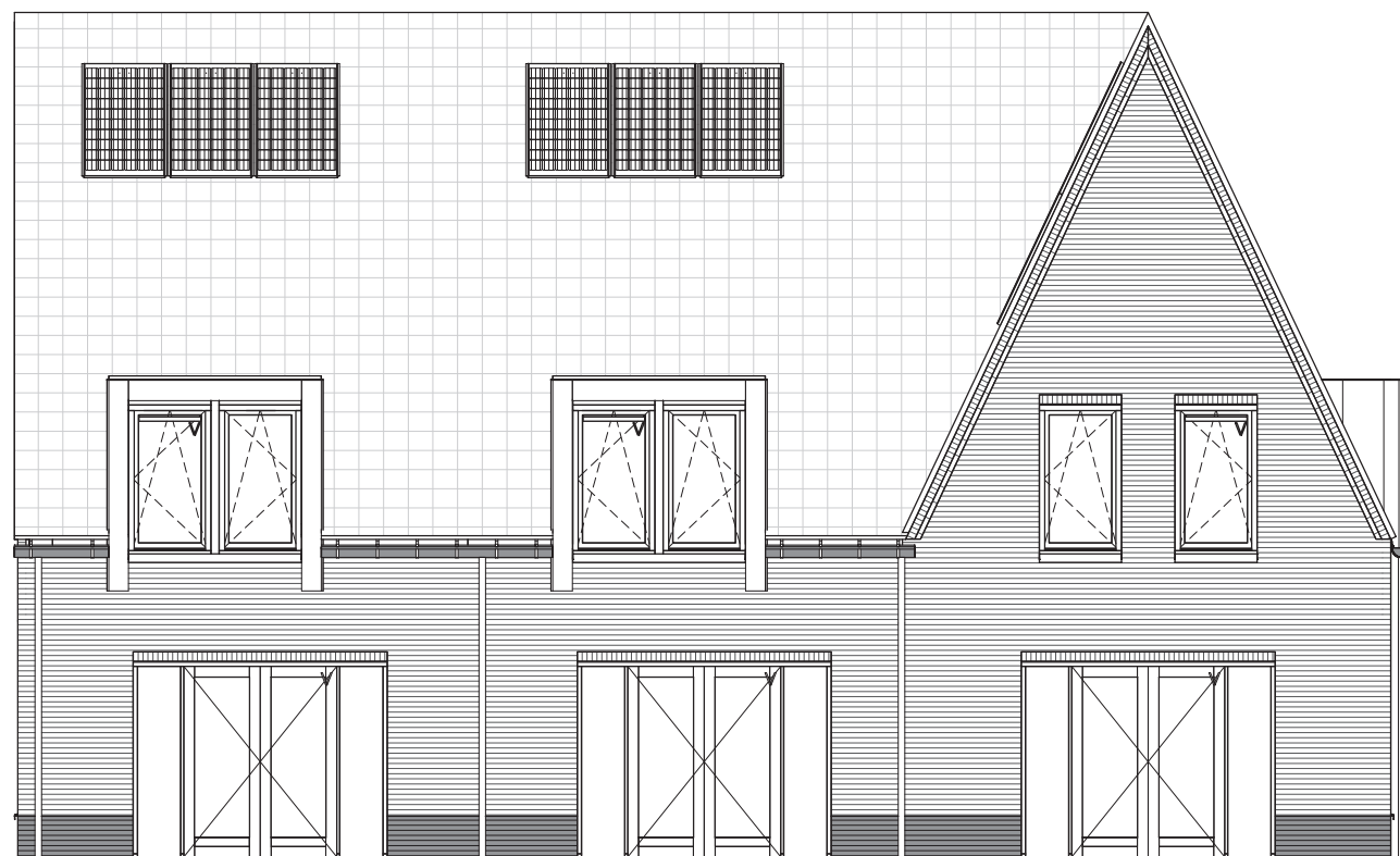
Voorgevel
