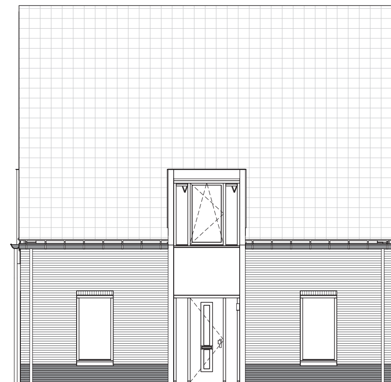
Rechtergevel
