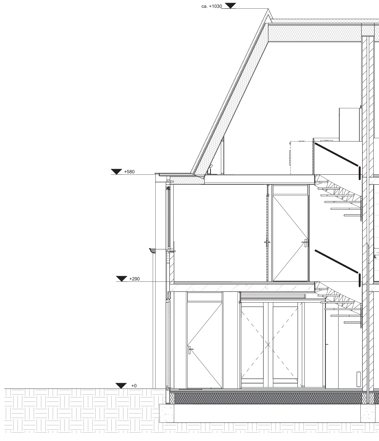
Doorsnede
