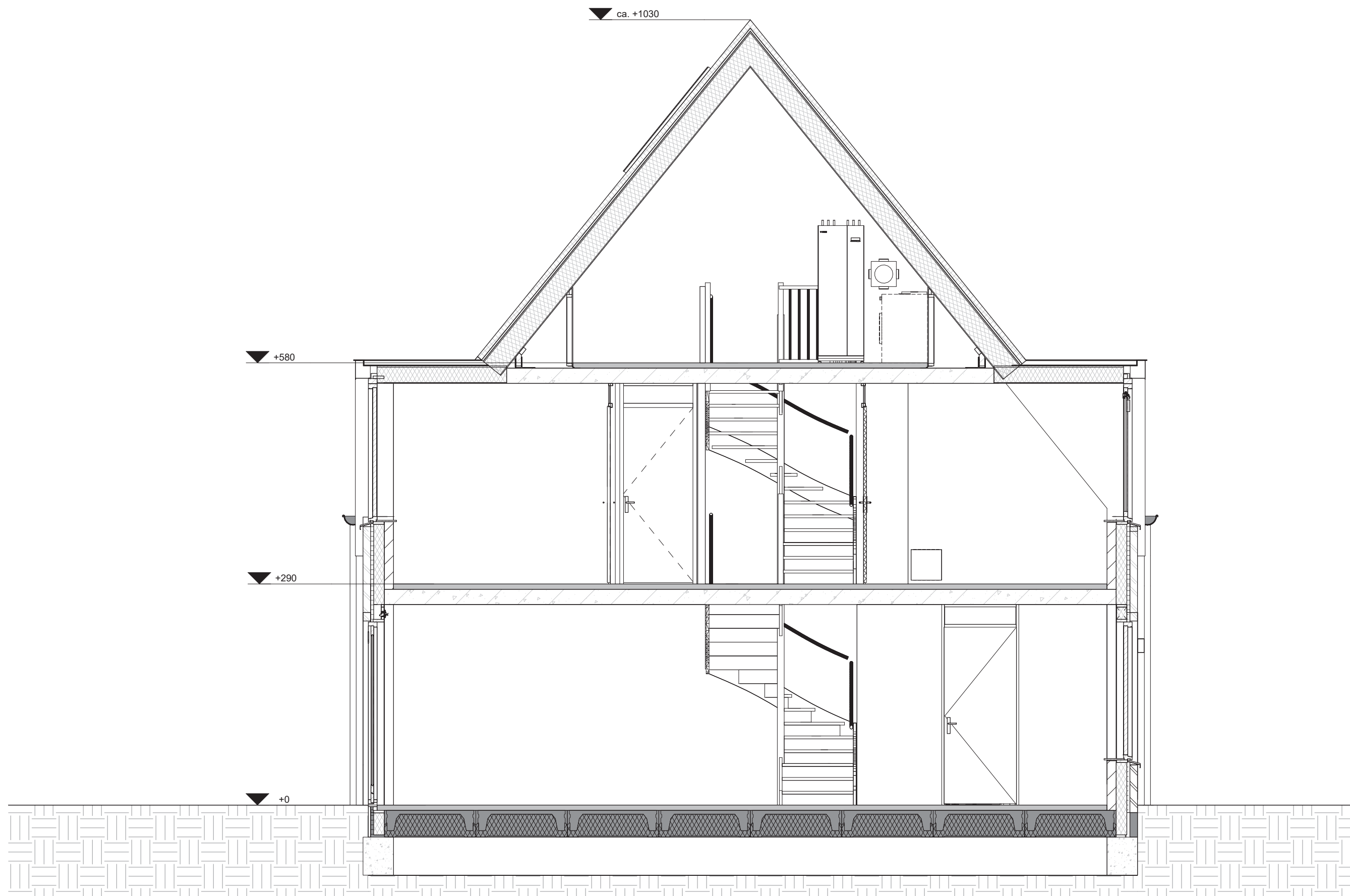
Doorsnede
